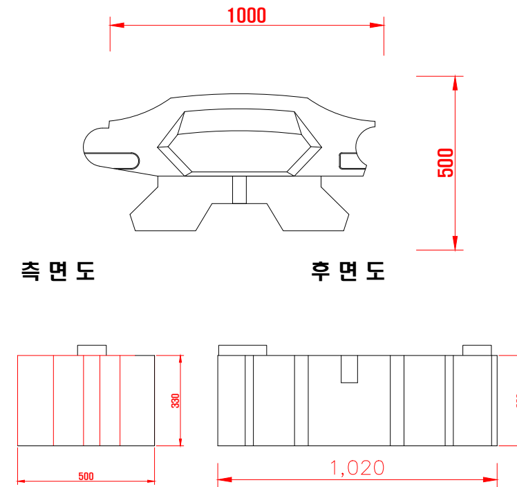
친환경 식생호안 옹벽 파도블럭 평면도
